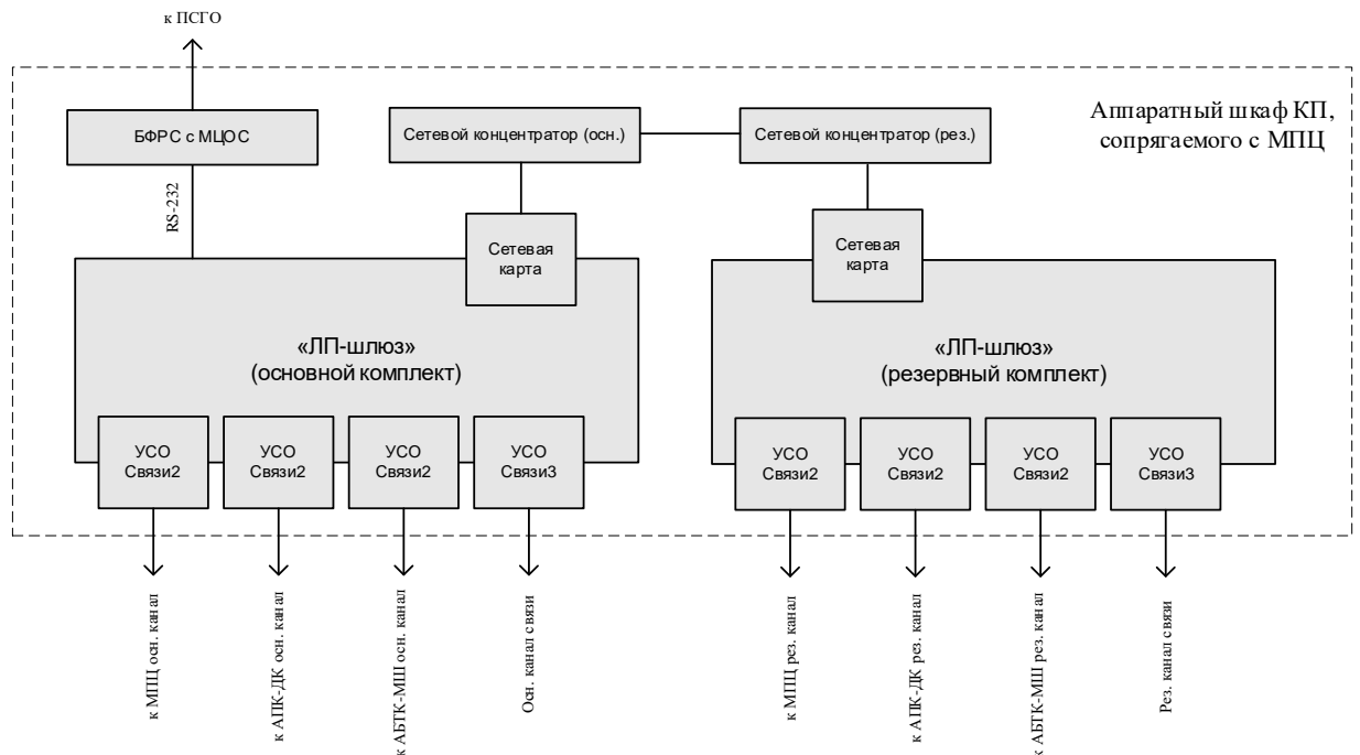
Рисунок 1 - Обобщенная структурная схема КП, сопрягаемого с МПЦ
